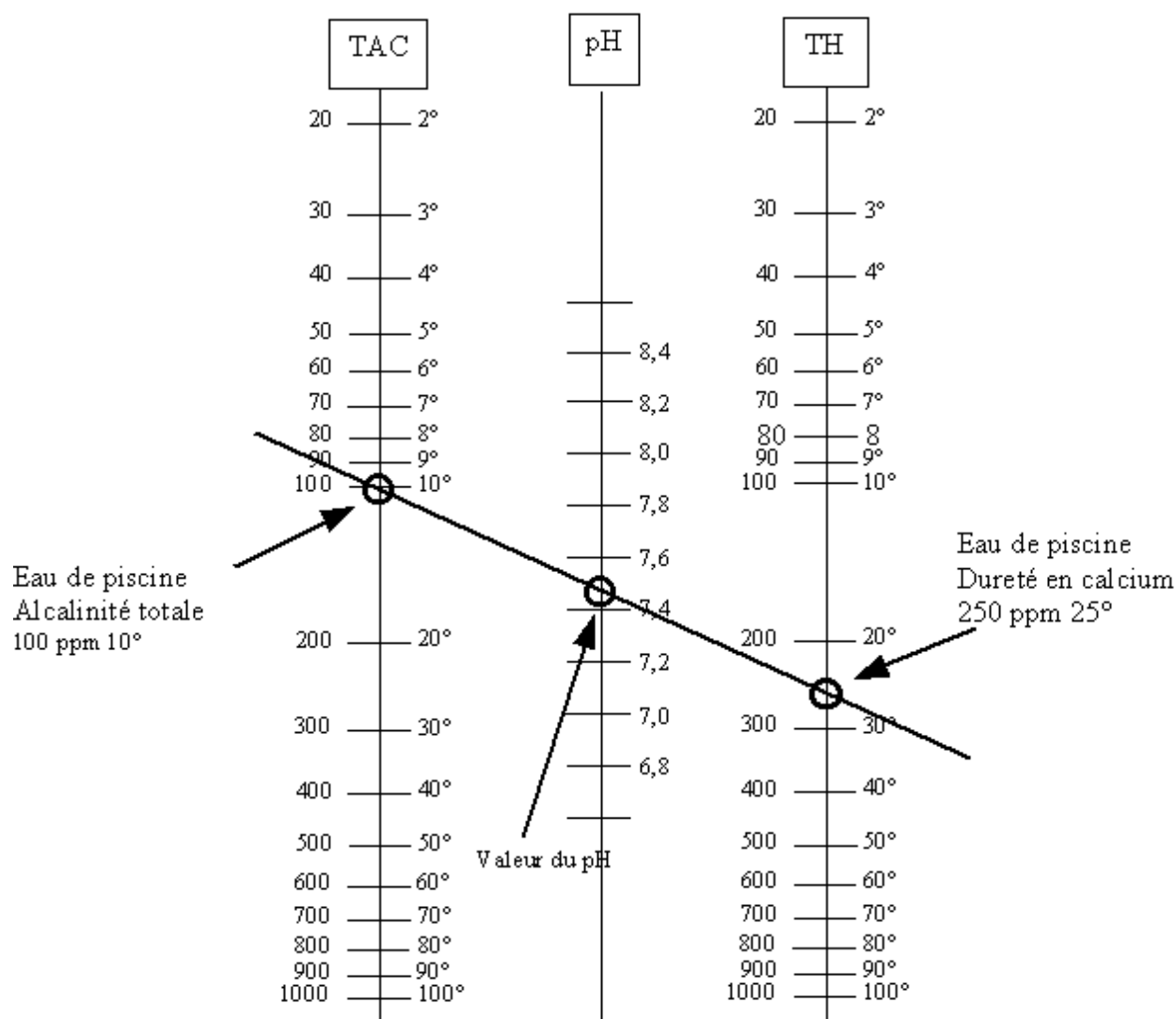
Diagramme d'équilibre de l'eau de piscine
